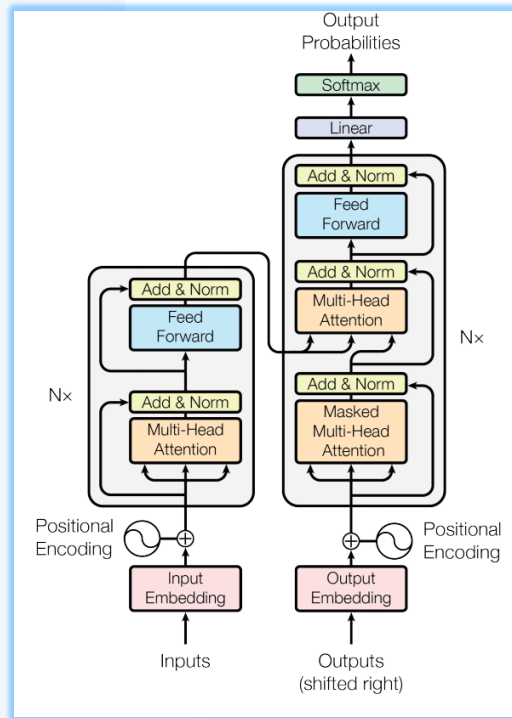
图27：Transformer模型架构如下所示
